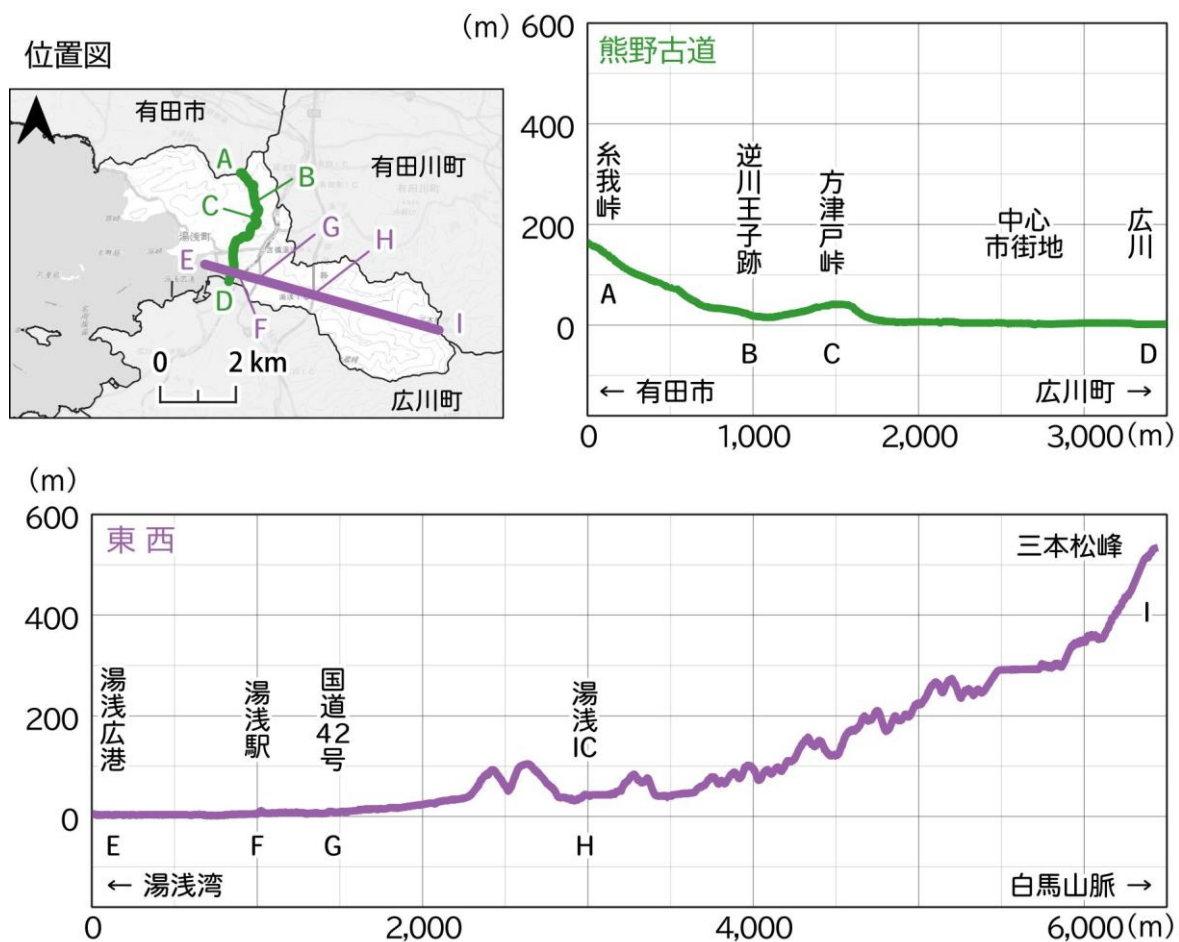
図 1-3 湯浅町の地形断面
