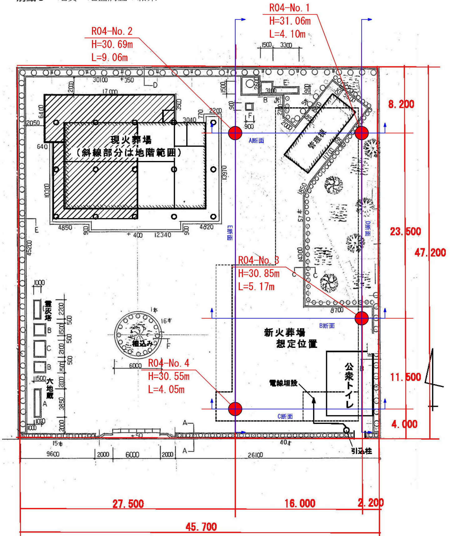
図 1.1.1 調査位置平面図 (S=1:200)
